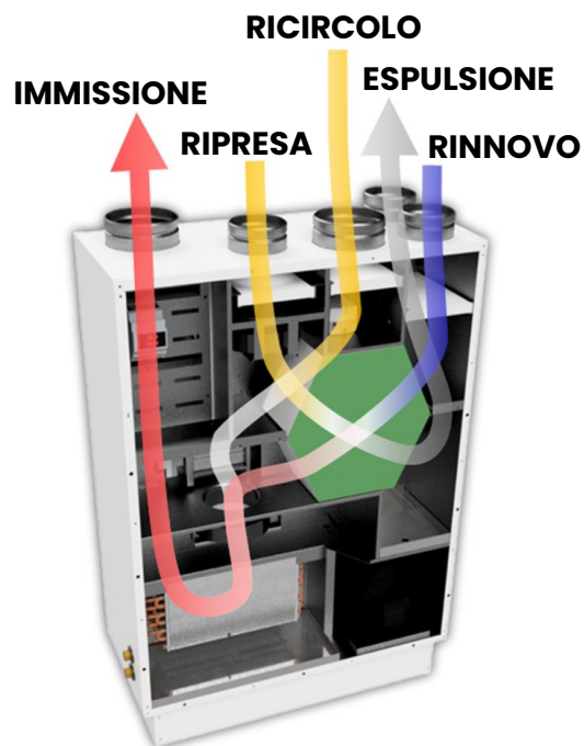
Flussi modalità ventilazione + ricircolo (deumidifica/integrazione)
